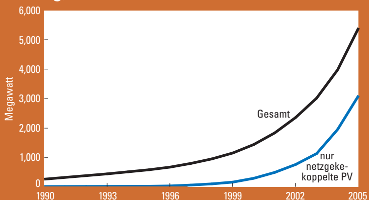
Abbildung 3. Photovoltaik, weltweit installierte Leistung, 1990–2005
