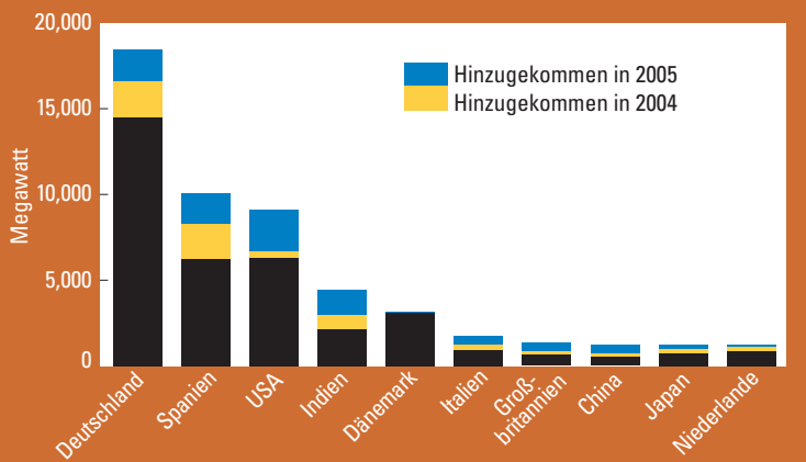
Abbildung 2. Windkraftleistung in den 10 führenden Ländern 2005
