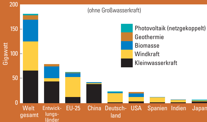
Abbildung 4. Kapazitäten für EE-Strom in Entwicklungsländern, der EU und den 6 führenden Ländern, 2005
